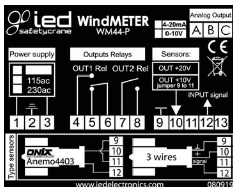
WM44-P. Etiqueta de conexionado
